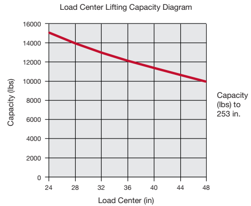
E70 (Simple Mast)
